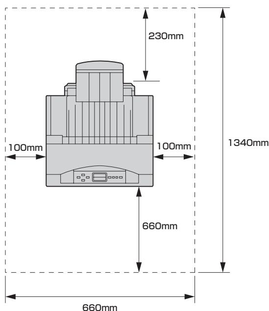
プリンター上面
