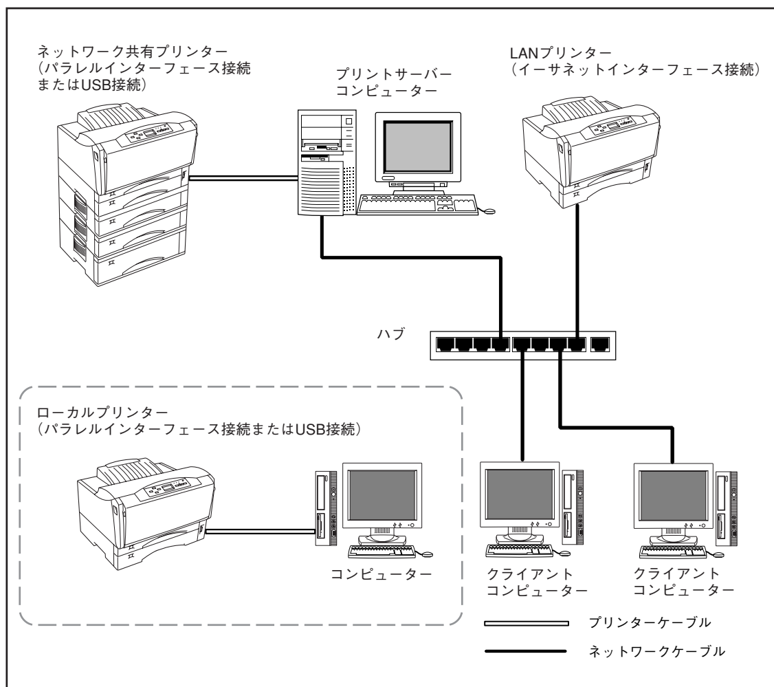
MultiWriter 2850Nの接続例
