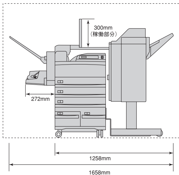
本体+オプション装着時 (大容量ホッパー+両面印刷ユニット+フェースアップトレイ +封筒フィーダー+フィニッシャー)
