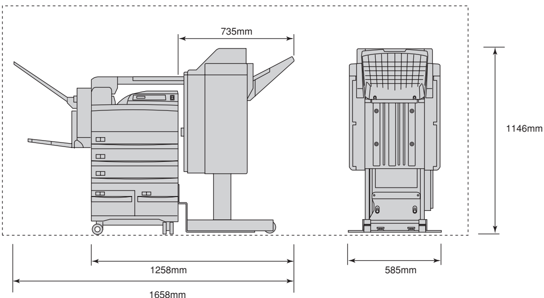
本体+オプション装着時 (大容量ホッパー+両面印刷ユニット+フェースアップトレイ+フィニッシャー)
