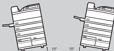
正面から見た図
