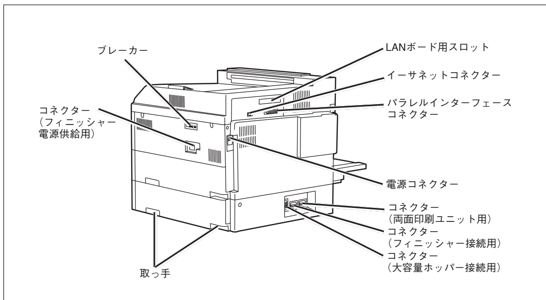
プリンター背面
