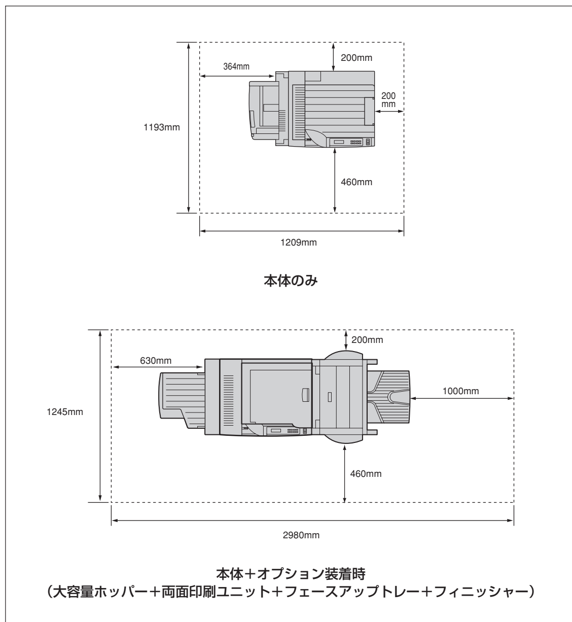
設置に必要なスペース(上から見たところ)
