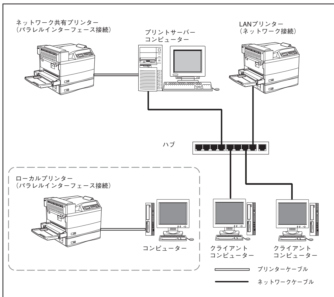
MultiWriter 4550の接続例
