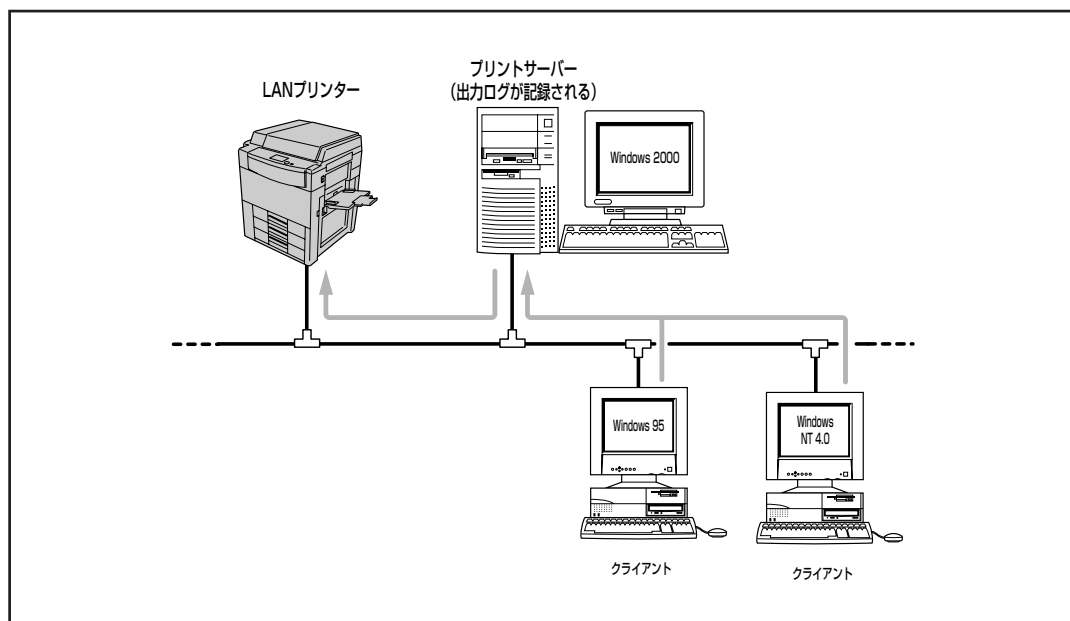
LANボードで接続されたプリンターの共有
